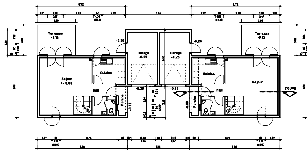
PLAN DE REZ DE CHAUSSEE
