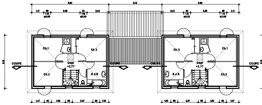
PLAN ETAGE
